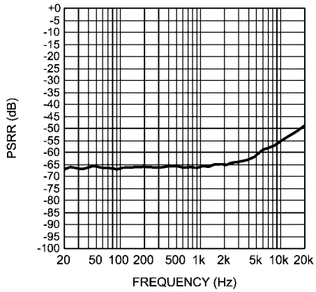
查询"LM49370RL"供应商 Loudspeaker PSRR vs Frequency AV_{DD} = 3.3V, 0dB\ AUX (AUX inputs terminated)
