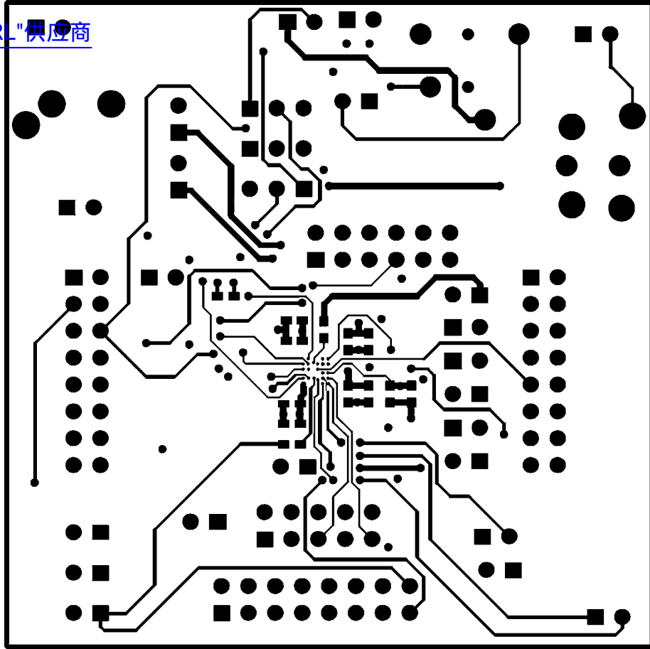
Bottom Layer
