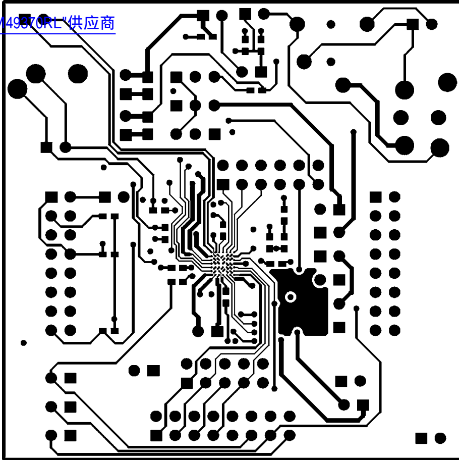
Top Layer
