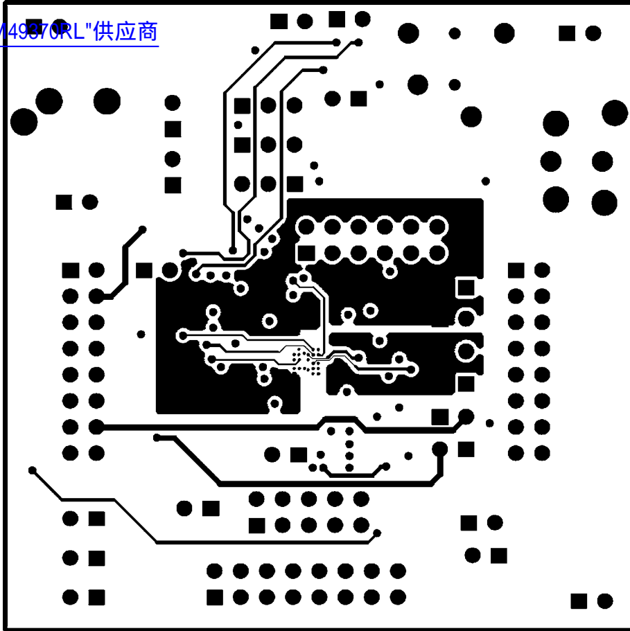
Mid Layer 2
