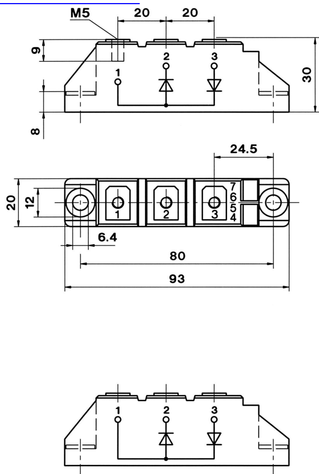
Case A 10 (SKKD)
