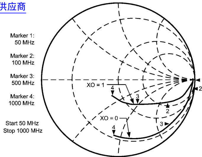
OSCin Input Impedance
