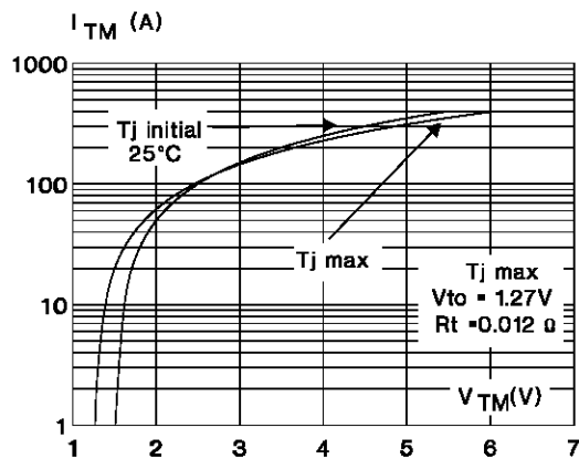
Fig11 : On-state characteristics (maximum values). 查询"BTW68-1000"供应商
