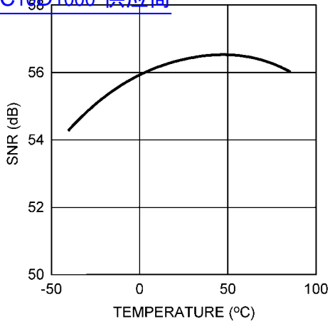
SNR vs. TEMPERATURE (ADC10D1000) 查询"ADC10D1000"供应商
