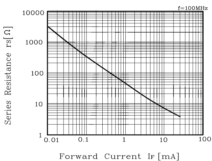
Fig. 4 r_s - I_F
