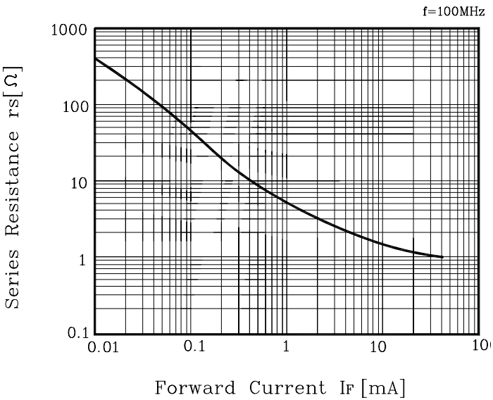
Fig. 2 r_s - I_F
