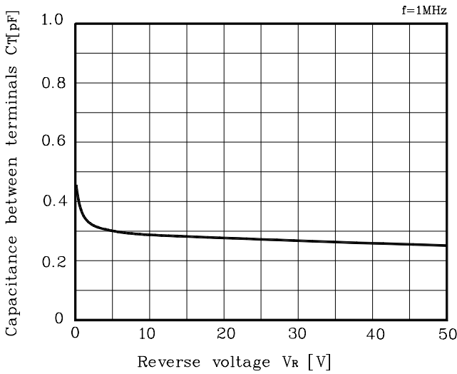
Fig. 1 C_T - V_R
