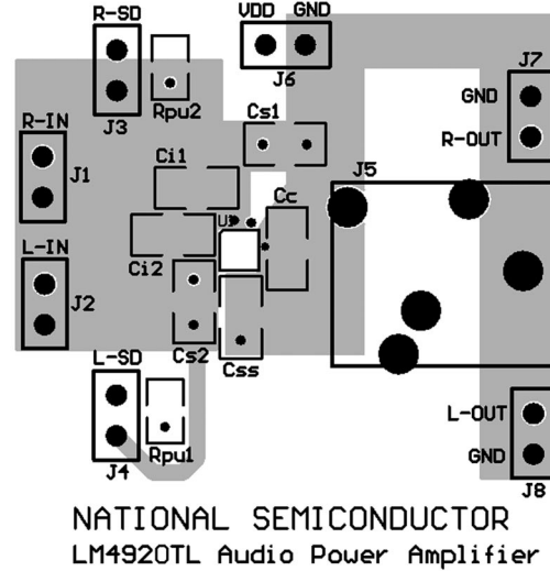
Bottom Layer
