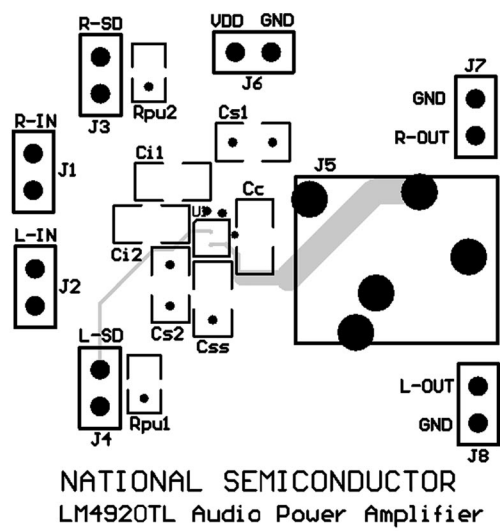
Mid Layer 1
