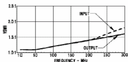
Input/Output VSWR
