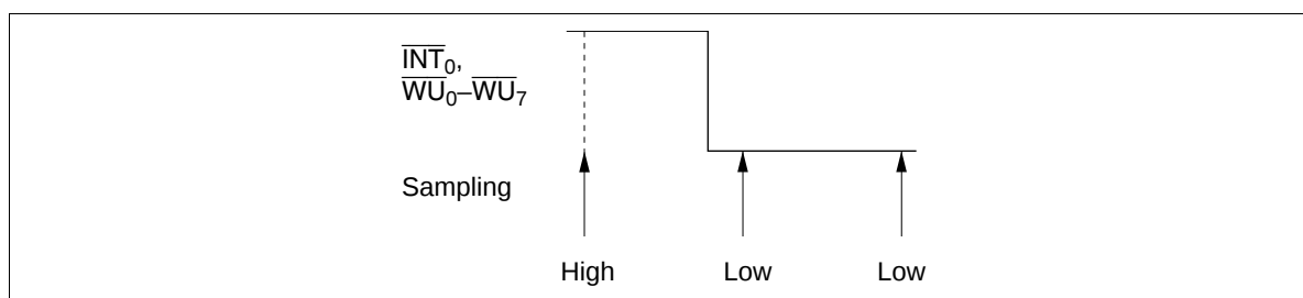
Figure 23 Edge Detection
