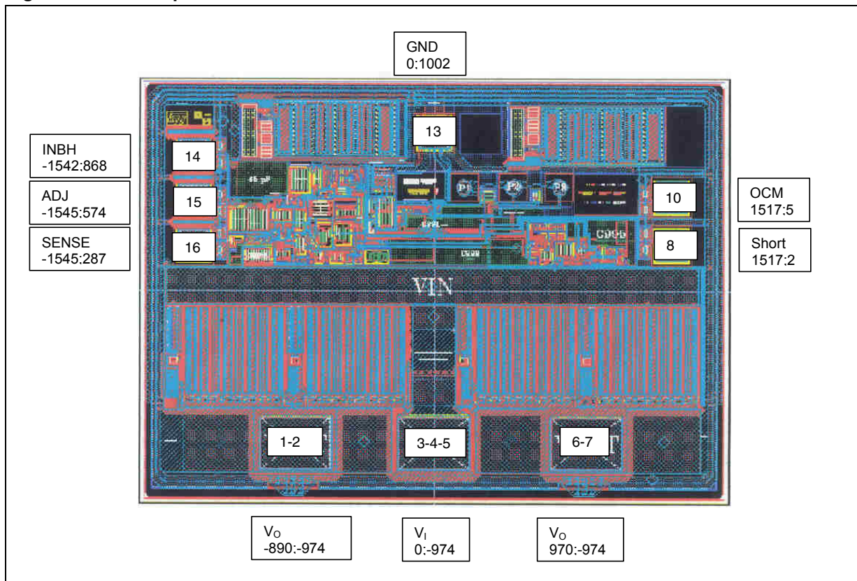
Figure 4. Die map
