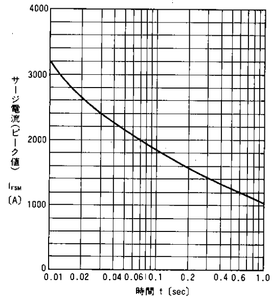
サージ電流
