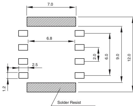
LAND PATTERNS(mm) 推奨ランド寸法
