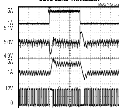
OUT5 LOAD TRANSIENT
