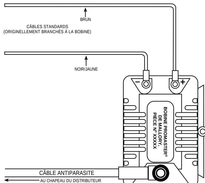
FIGURE 5 ALLUMAGE ÉLECTRONIQUE CHRYSLER
