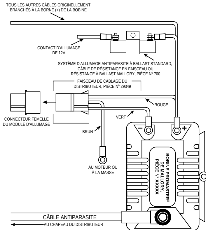
FIGURE 3 ALLUMAGE ÉLECTRONIQUE MALLORY ALLUMAGE ÉLECTRONIQUE UNILITE® ALLUMAGE MAGNÉTIQUE SANS RUPTEUR ET AVANCE À ALLUMAGE ÉLECTRONIQUE
