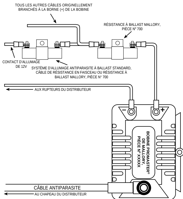
FIGURE 2 ALLUMAGE DU PLOT DE CONTACT CONTACTS SIMPLES OU DOUBLES SCHEMA POUR LE CÂBLAGE DE LA BOBINE MARK II DE VOLTMASTER®)
