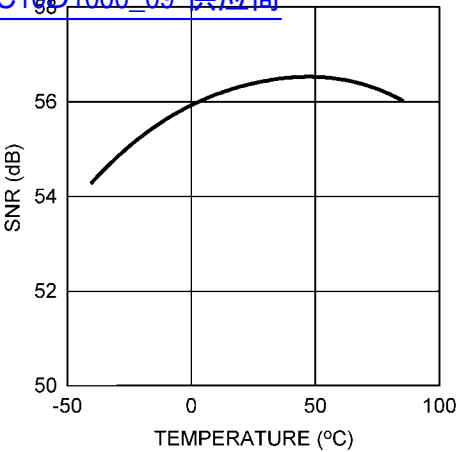
SNR vs. TEMPERATURE (ADC10D1000) 查询"ADC10D1000_09"供应商
