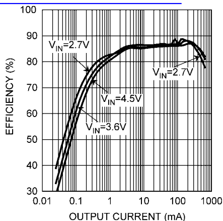
Efficiency vs. Output Current 查询"LM3677" 1.5V 供应商
