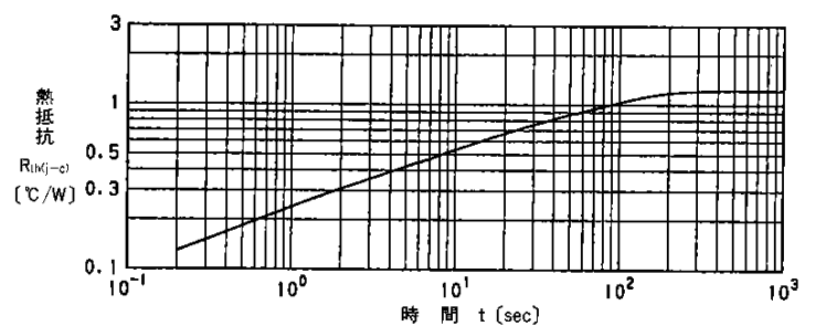
過渡熱抵抗(ツェナーダイオード)特性 Transient Thermal Resistance (Zener Diode)
