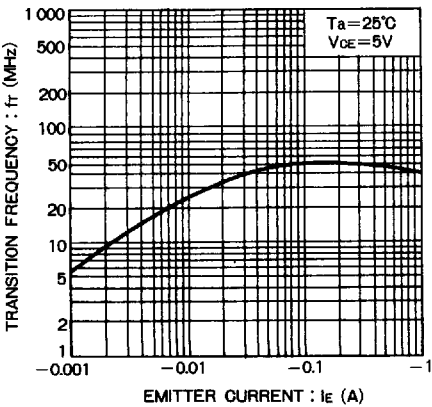
Fig.9 利得帯域幅-エミッタ電流特性
