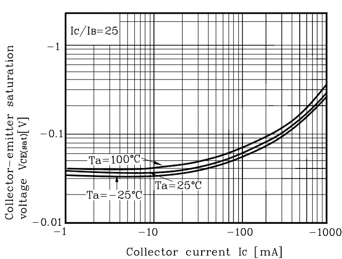
Fig. 5 V_{CE(SAT)} - I_c
