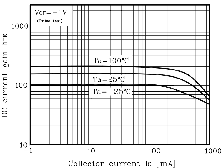
Fig. 4 h_{FE} - I_c
