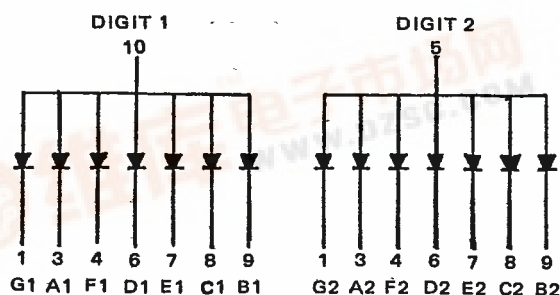
CS-322 COMMON ANODE
