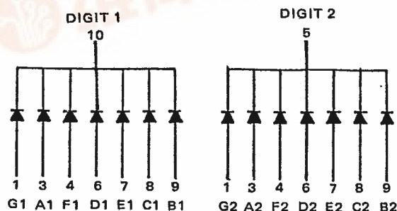
CS-323 COMMON CATHODE
