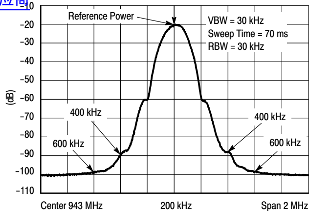
Figure 24. EDGE Spectrum
