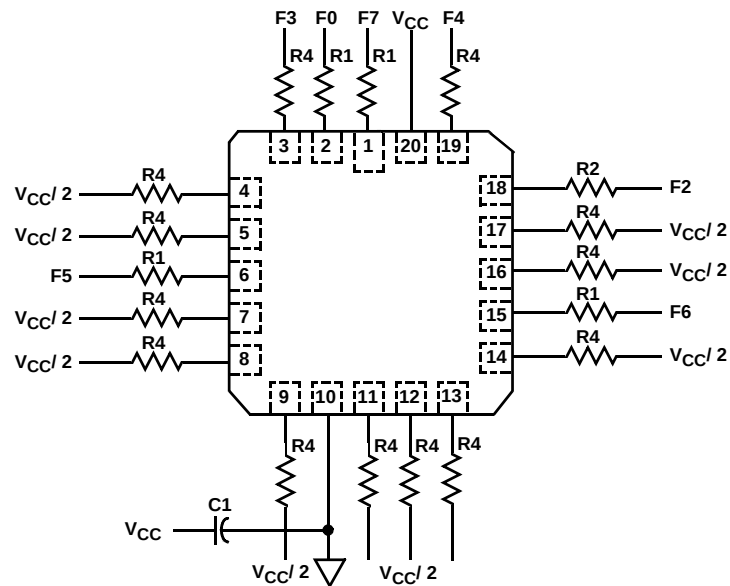
MR82C88 CLCC
