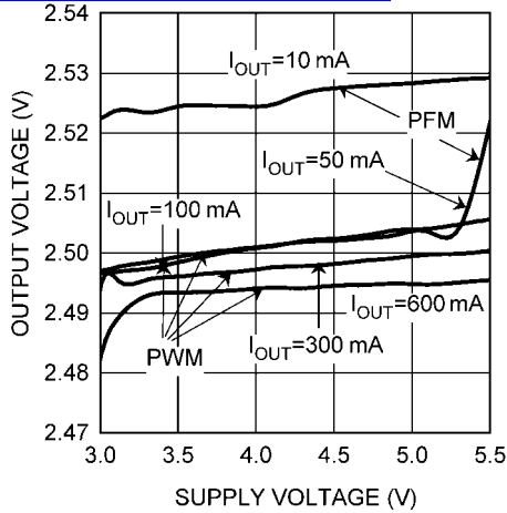
Output Voltage vs. Supply Voltage 查询"LM3677" (V OUT = 1.32V) 应用
