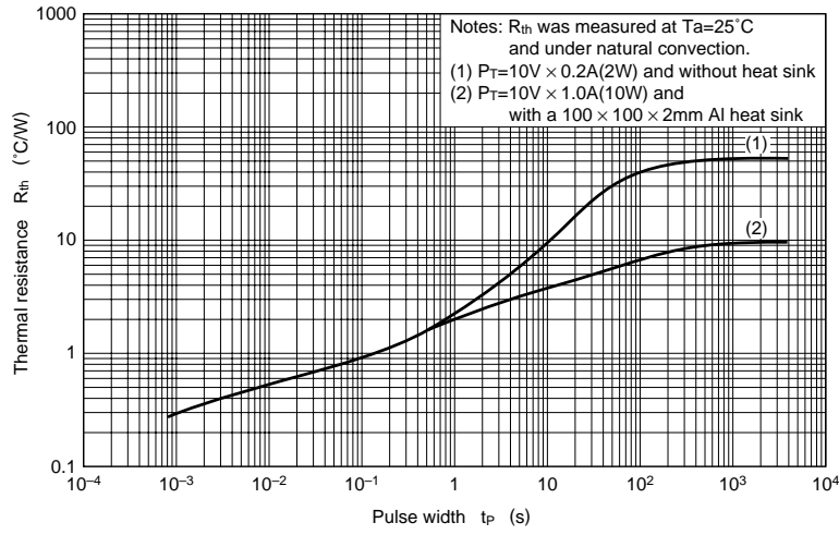
R_{th} - t_p
