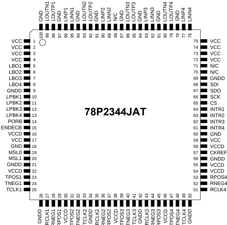
100-pin TQFP (JEDEC LQFP)
