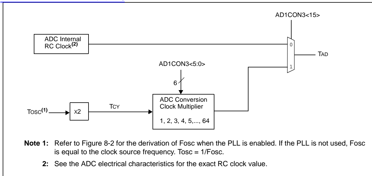
查閱 dsPIC33FJ64GPX02 中文資料 FIGURE 21-3: ADC CONVERSION CLOCK PERIOD BLOCK DIAGRAM
