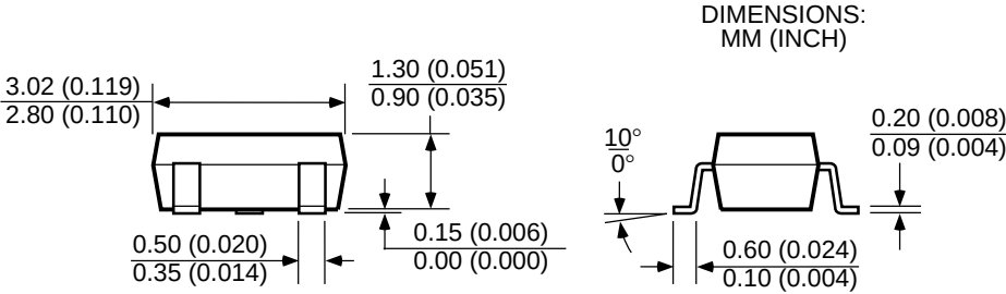
SOT-23-5 (M)
