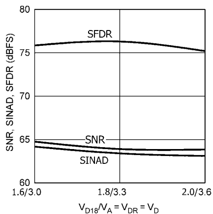
SNR, SINAD, SFDR vs. V_{SUPPLY}
