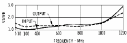
VSWR
