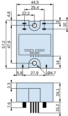
Dimensions
