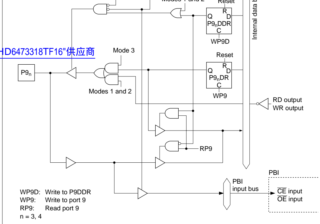
Figure C.9 (d) Port 9 Block Diagram (Pins P9 3 , P9 4 )
