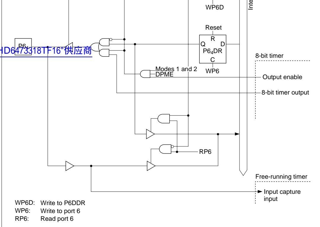
Figure C.6 (d) Port 6 Block Diagram (Pin P6 4 )
