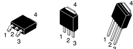
CASE 369AA DPAK (Bent Lead) STYLE 2
