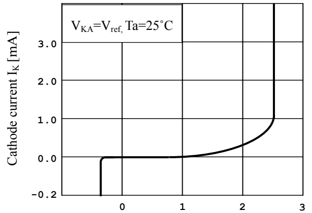
Fig.5 I_K vs V_{KA} (2)
