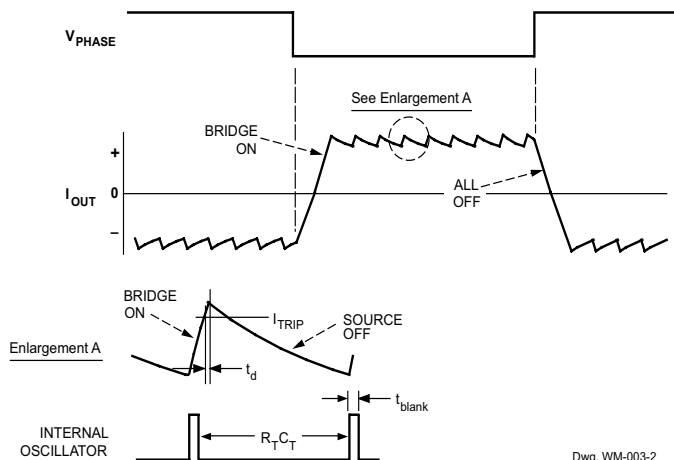
Dwg. WM-003-2
