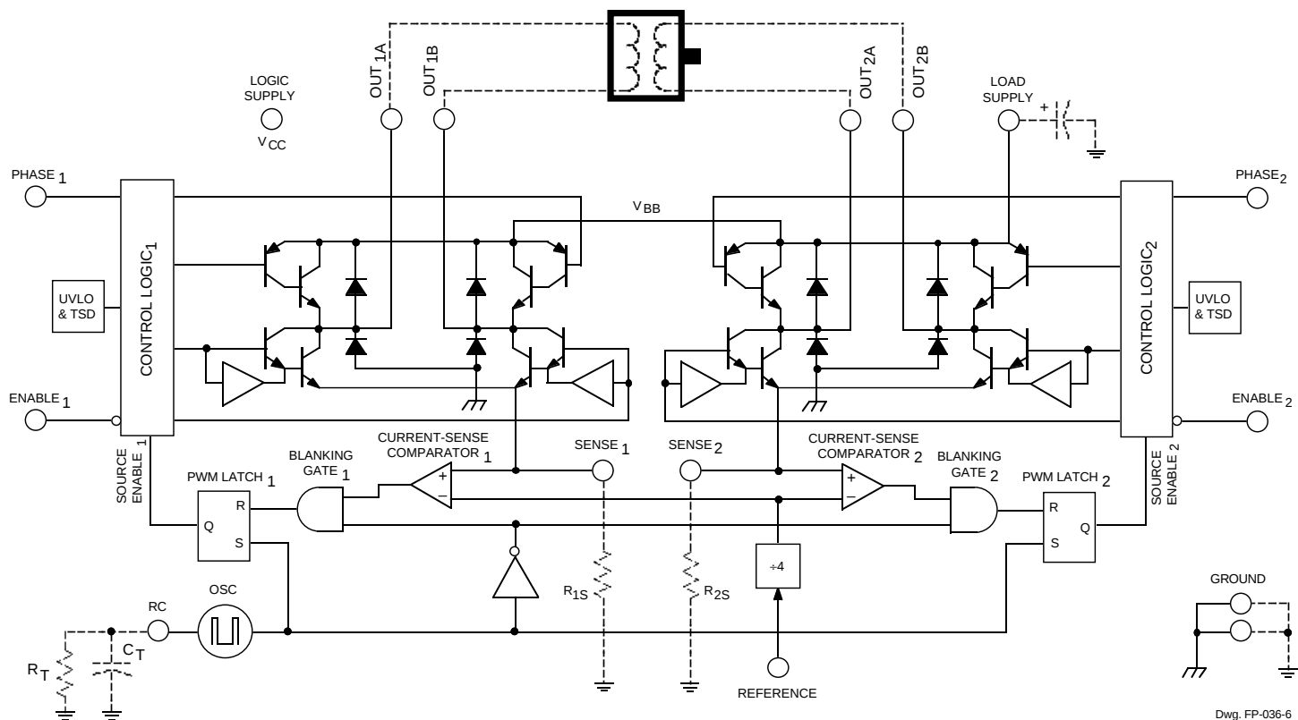
Dwg. FP-036-6
