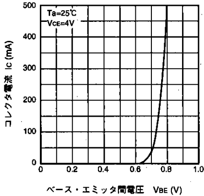
エミッタ接地伝達特性 (1)
