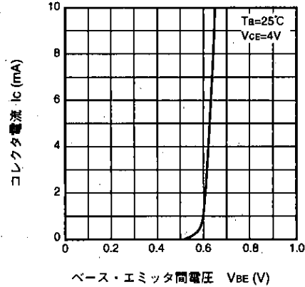
エミッタ接地伝達特性 (2)
