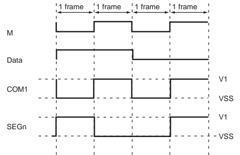
(d) Waveform with static output
