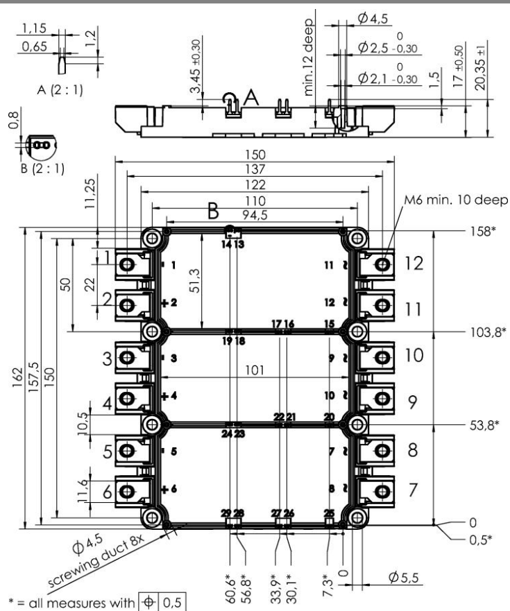
Case SEMiX 33c
