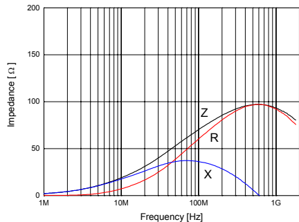
SHB-1T1005-700J
