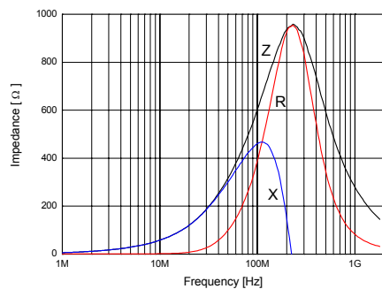
SHB-1M1005-601J
