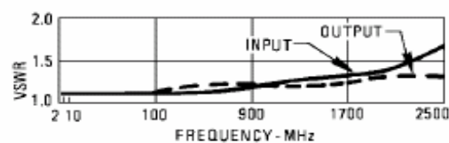
VSWR
