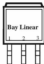
TO-263-3 (S)
