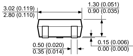
SOT-23-5 (M)
