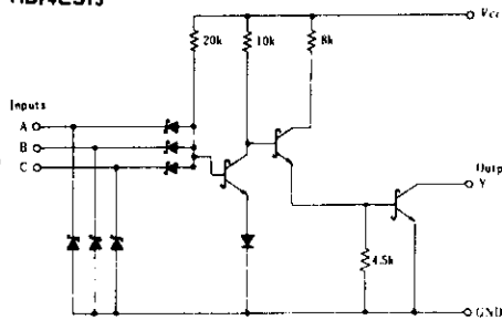
HD74LS15
