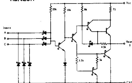
HD74LS11
