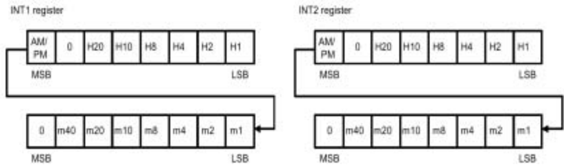
图 8 实时时钟 INT1 和 INT2 寄存器为报警时间数据
