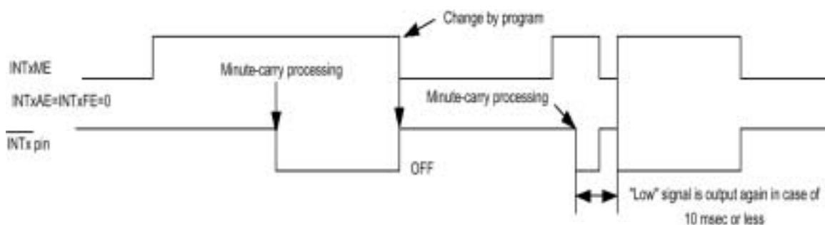
图 20 实时时钟每分钟边沿中断输出
