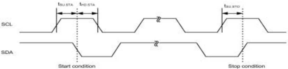
图 3 实时时钟的串行接口
