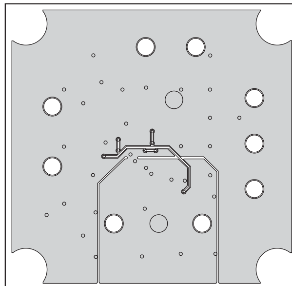
Bottom Side(Layer 4)
