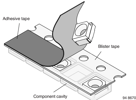
Fig. 9 - Blister Tape
