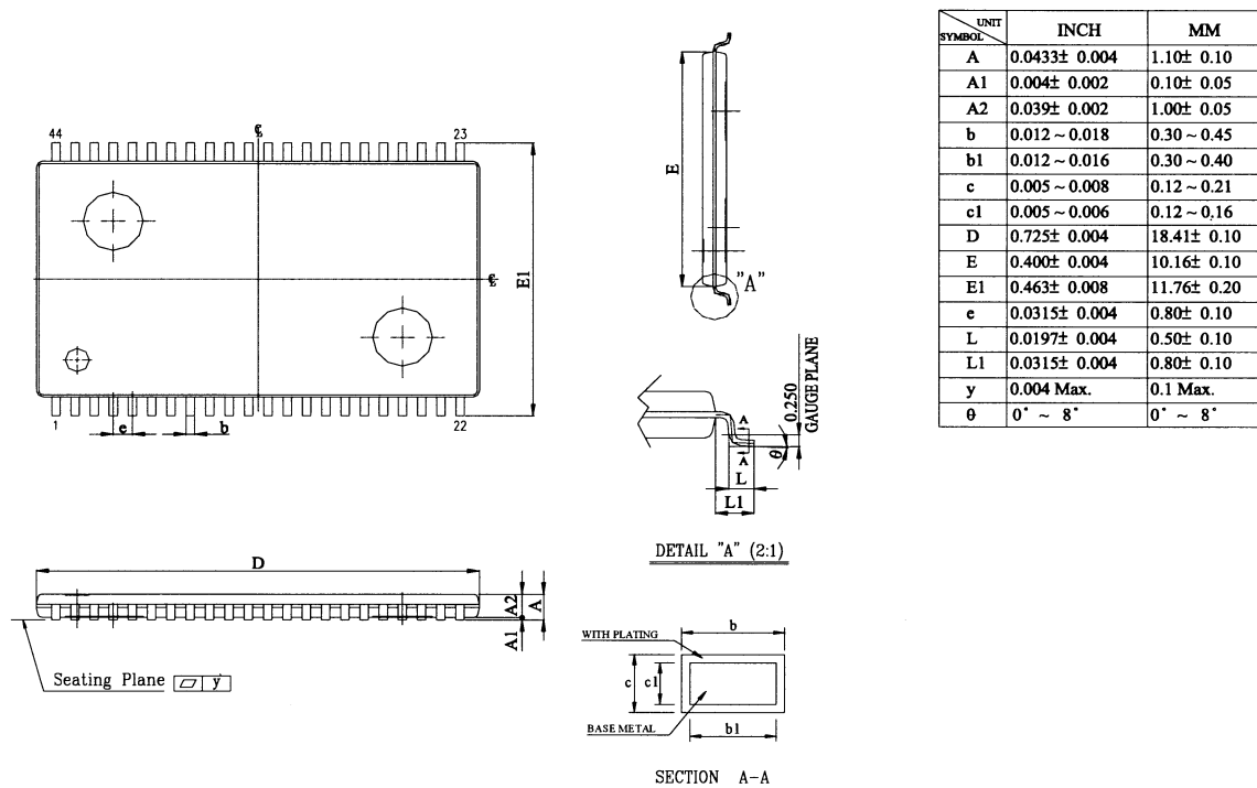
TSOP II-44
