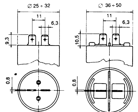
Fig. 2 Faston semplice 6,3 x 0,8 mm Fig. 2 Single tag 6.3 x 0.8 mm
