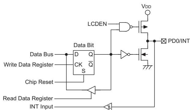
PD0 Input/Output Port
