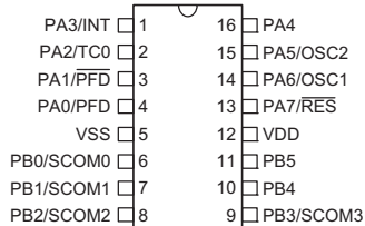
HT48R064 HT48R065 16 DIP-A/NSOP-A
