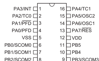
HT48R066 16 DIP-A/NSOP-A
