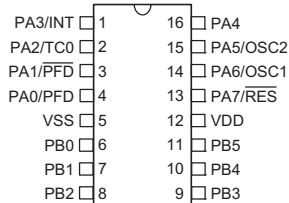
HT48R063 16 DIP-A/NSOP-A
